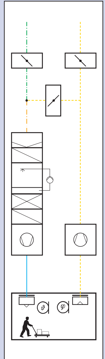
Beispielhafte Darstellung einer RLT-Anlage nach DIN 1946 Teil 1
